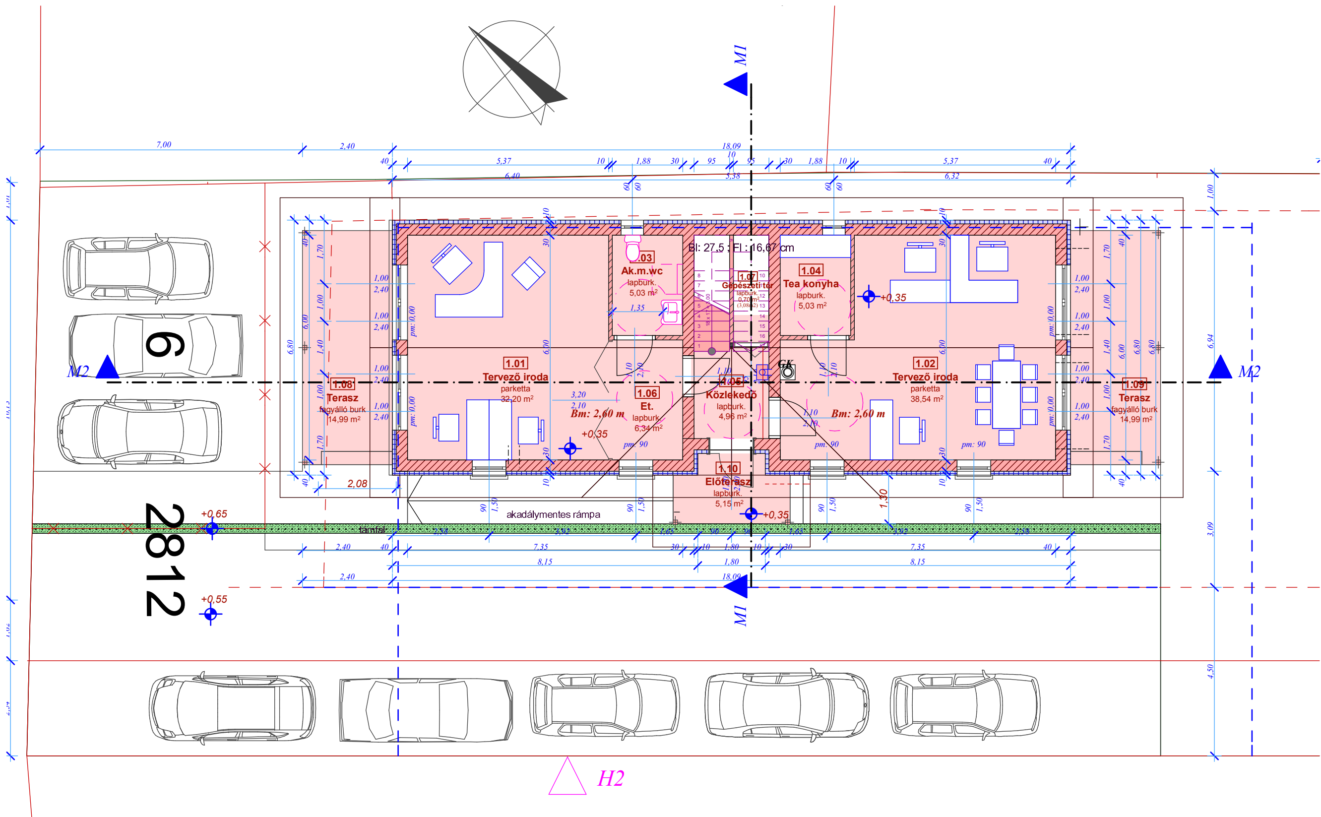
0. Földszint 1:100
